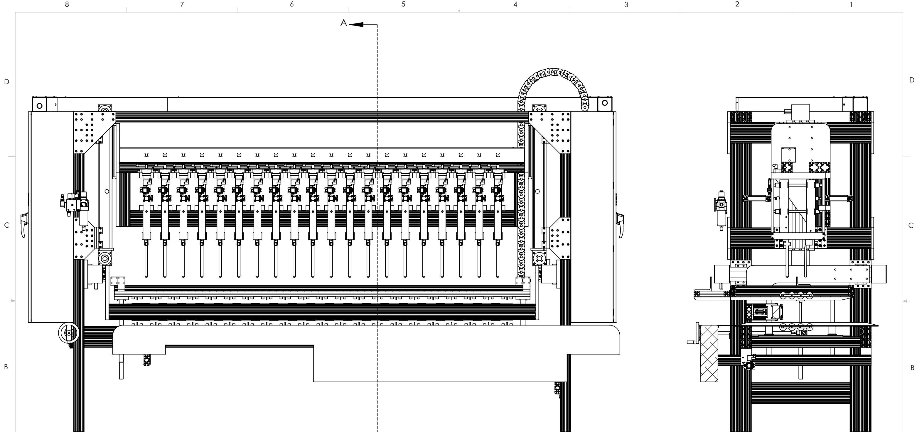
SECTION A-A SCALE 1 : 16
